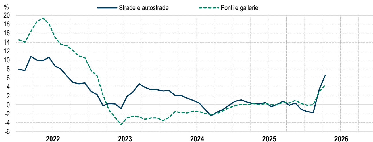
FIGURA 10. PREZZI ALLA PRODUZIONE DELLE COSTRUZIONI. STRADE E AUTOSTRADE, PONTI E GALLERIE, VARIAZIONI PERCENTUALI TENDENZIALI
