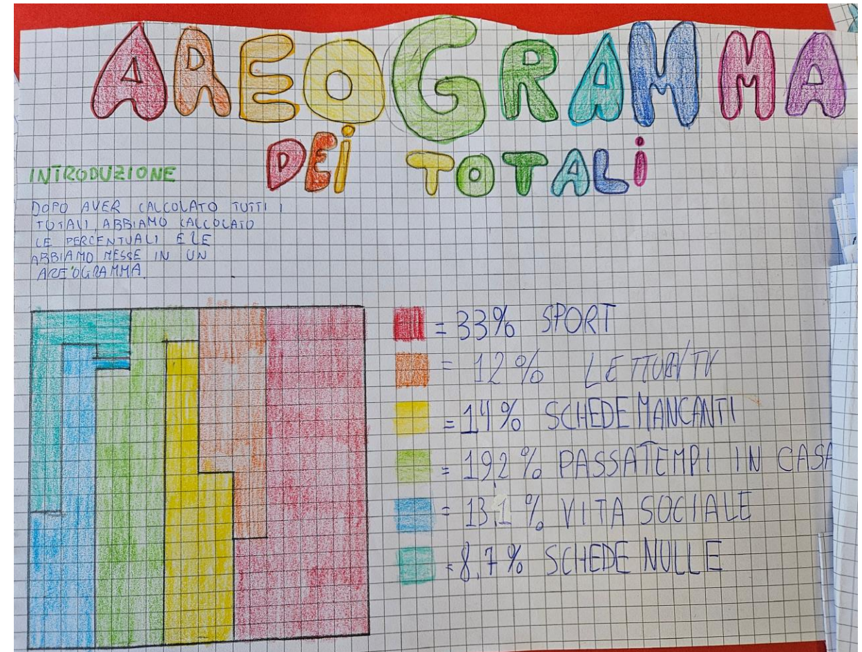
Areogramma
