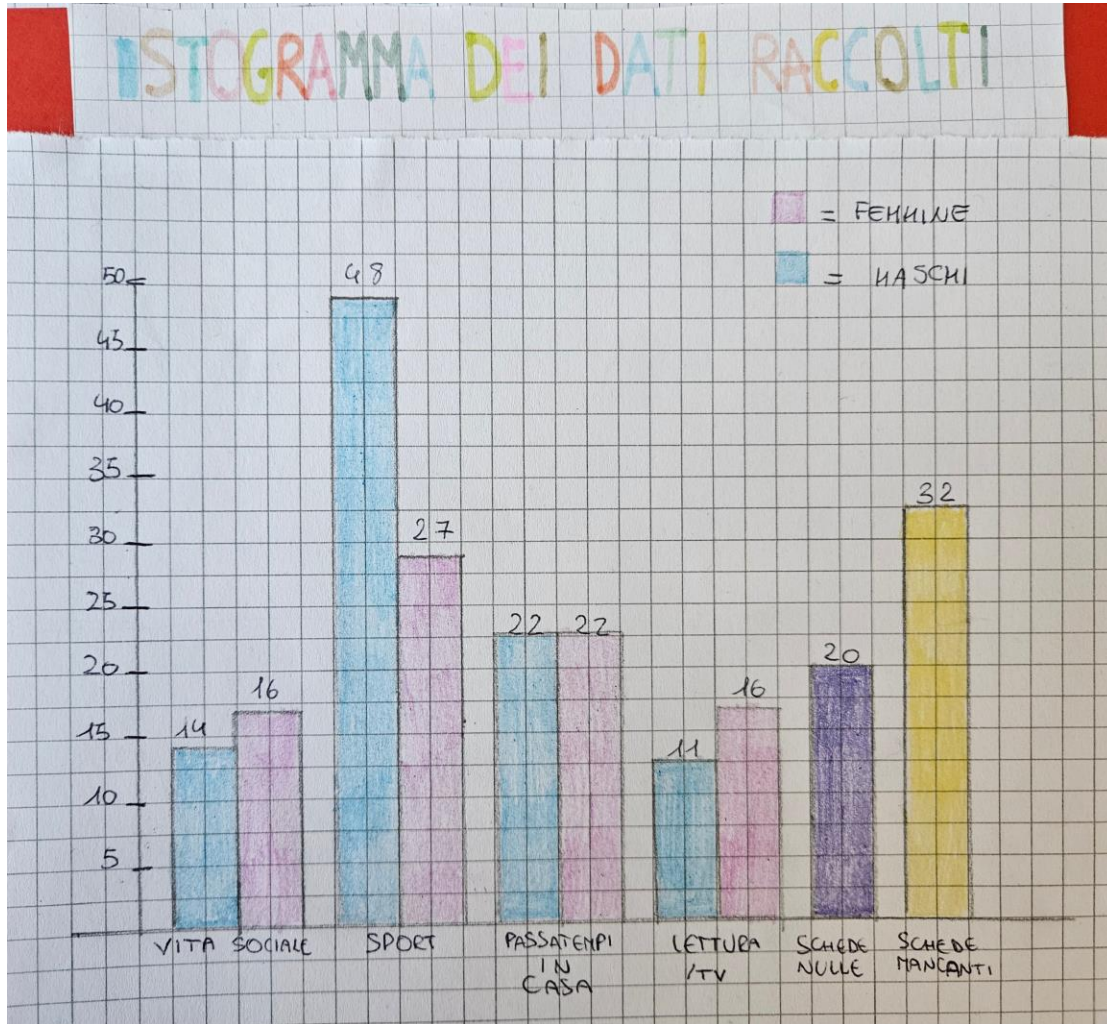
Istogramma
