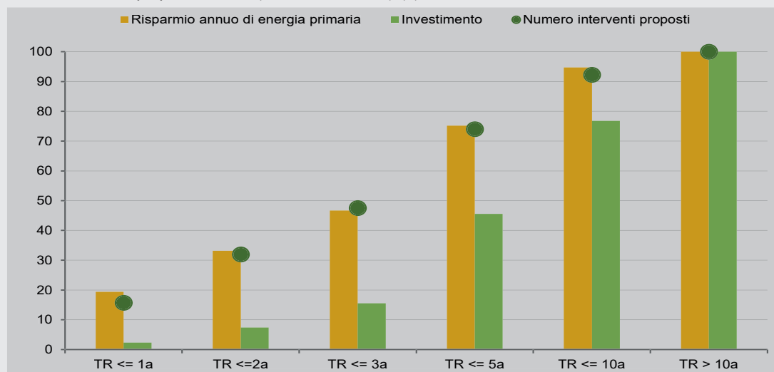
Figura 1 - Risparmio annuo di energia primaria, investimenti e numero di interventi proposti per tempo di ritorno (TR). Anno 2023 (valori percentuali) (a)
