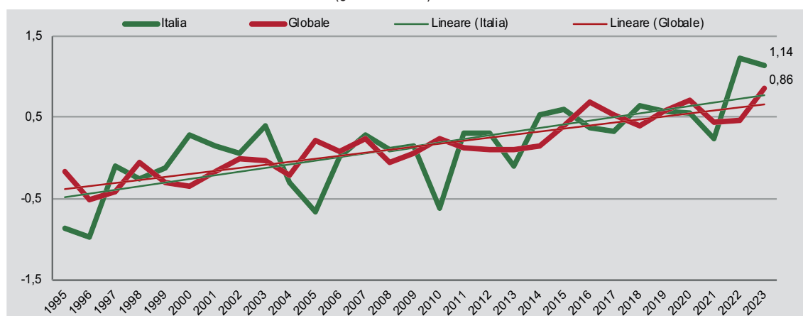
Figura 13.3 - Anomalie di temperatura media sulla terraferma a livello globale e in Italia, rispetto ai valori climatologici normali 1991-2020. Anni 1995-2023 (gradi Celsius)
