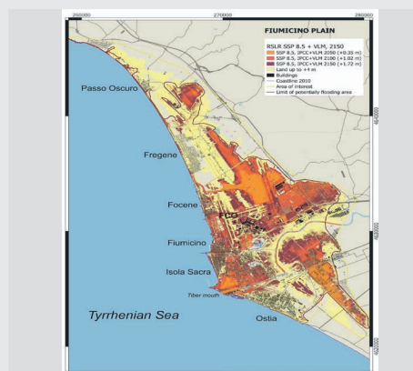
Figura 1b - Scenario di inondazione per la costa di Fiumicino
