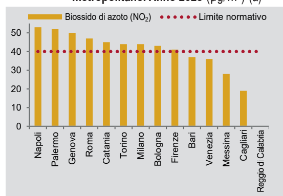
Figura 11.4 - Concentrazione media annua di biossido di azoto nei capoluoghi delle Città metropolitane. Anno 2023 (µg/m³) (a)
