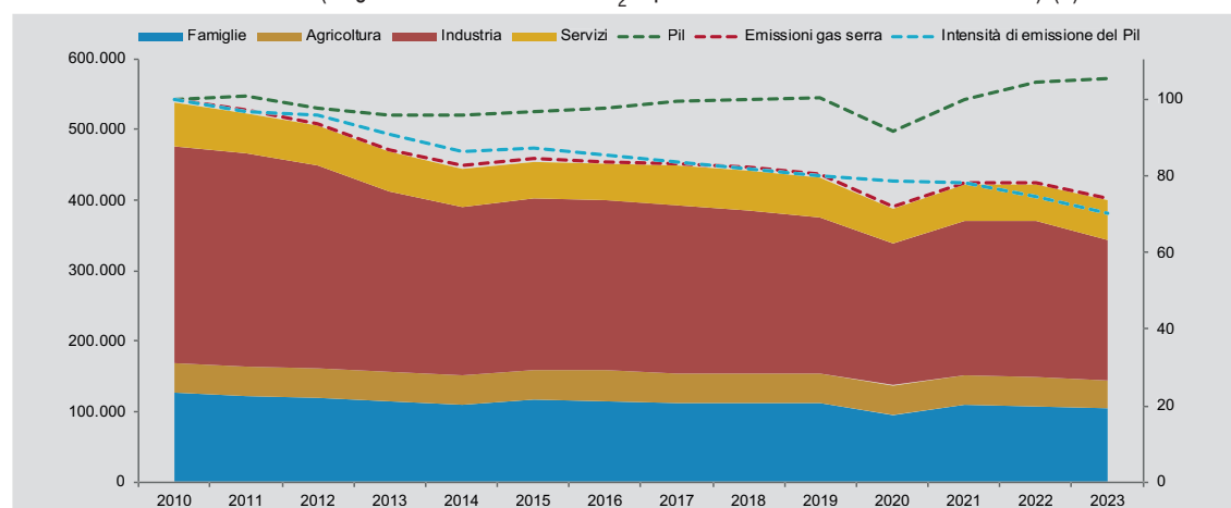
Figura 13.1 - Gas serra totali secondo i conti nazionali delle emissioni atmosferiche, Pil e intensità di emissione. Anni 2010-2023 (migliaia di tonnellate di CO 2 equivalente e numeri indici 2010=100) (a)
