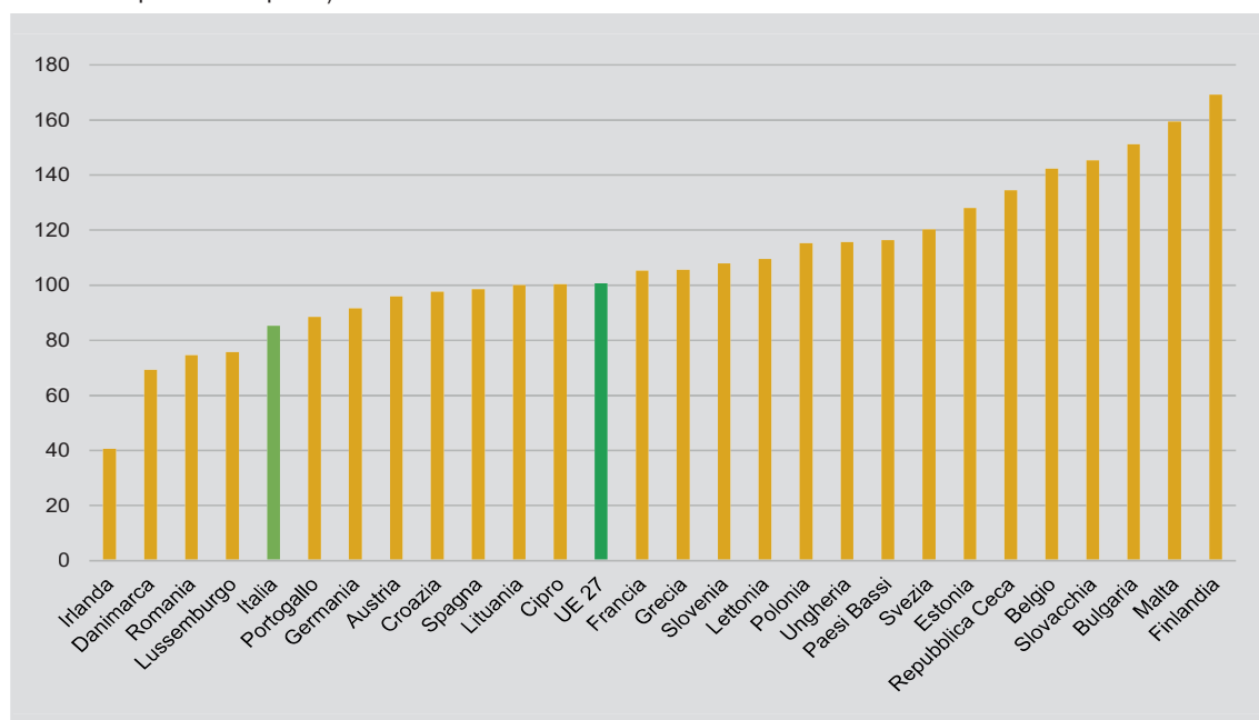
Figura 7.2 - Intensità energetica, per Paese. Anno 2021 (tonnellate equivalenti petrolio per milione di euro a parità di potere d'acquisto)
