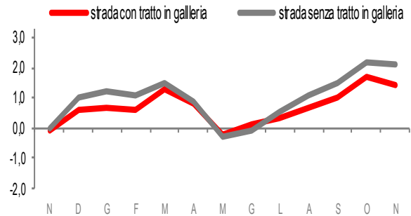
COSTO DI COSTRUZIONE DI TRONCHI STRADALI. Novembre 2016 - novembre 2017, variazioni percentuali tendenziali
