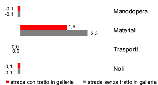
COSTO DI COSTRUZIONE DI TRONCHI STRADALI. Novembre 2017, contributi alla variazione tendenziale degli indici per gruppi di costo, punti percentuali
