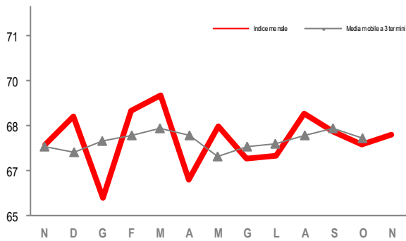
PRODUZIONE NELLE COSTRUZIONI. Novembre 2016 - novembre 2017, indice destagionalizzato e media mobile a tre termini
