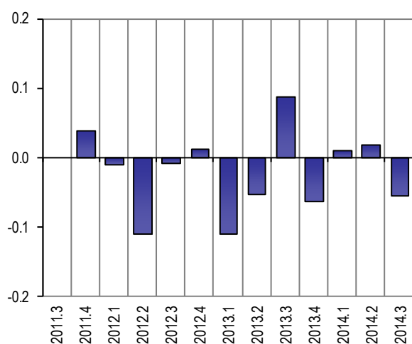
Revisioni in termini congiunturali della stima preliminare del PIL (differenze tra la prima stima dei conti trimestrali e la stima preliminare). Dati destagionalizzati. Periodo 2011:3- 2014:3
