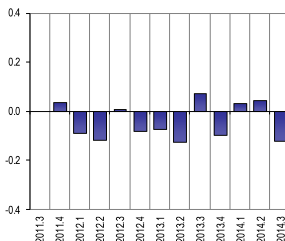
Revisioni in termini tendenziali della stima preliminare del PIL (differenze tra la prima stima dei conti trimestrali e la stima preliminare). Dati destagionalizzati. Periodo 2011:3- 2014:3
