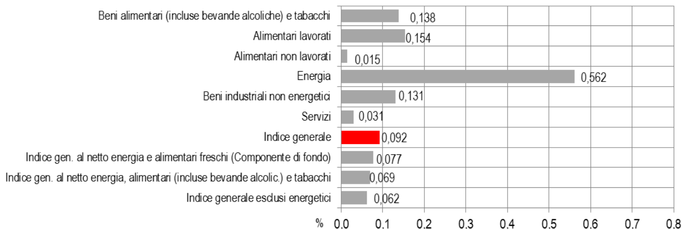
FIGURA 1. REVISIONE MEDIA ASSOLUTA DELLE STIME PRELIMINARI DEI TASSI TENDENZIALI DEGLI INDICI IPCA Settembre 2021 – settembre 2022, punti percentuali
