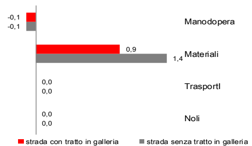
COSTO DI COSTRUZIONE DI TRONCHI STRADALI. Gennaio 2017, contributi alla variazione tendenziale degli indici per gruppi di costo, punti percentuali
