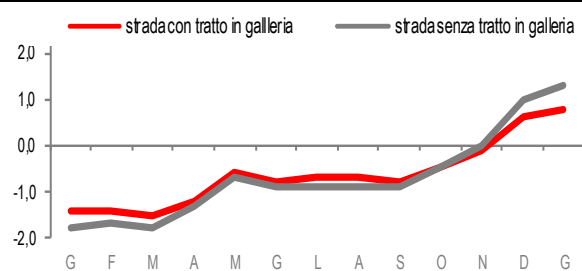
COSTO DI COSTRUZIONE DI TRONCHI STRADALI. Gennaio 2016 - gennaio 2017, variazioni percentuali tendenziali
