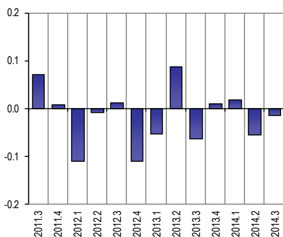
Revisioni in termini congiunturali della stima preliminare del PIL (differenze tra la prima stima dei conti trimestrali e la stima preliminare). Dati destagionalizzati. Periodo 2011:2- 2014:4
