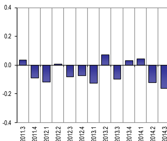
Revisioni in termini tendenziali della stima preliminare del PIL (differenze tra la prima stima dei conti trimestrali e la stima preliminare). Dati destagionalizzati. Periodo 2011:2- 2014:4
