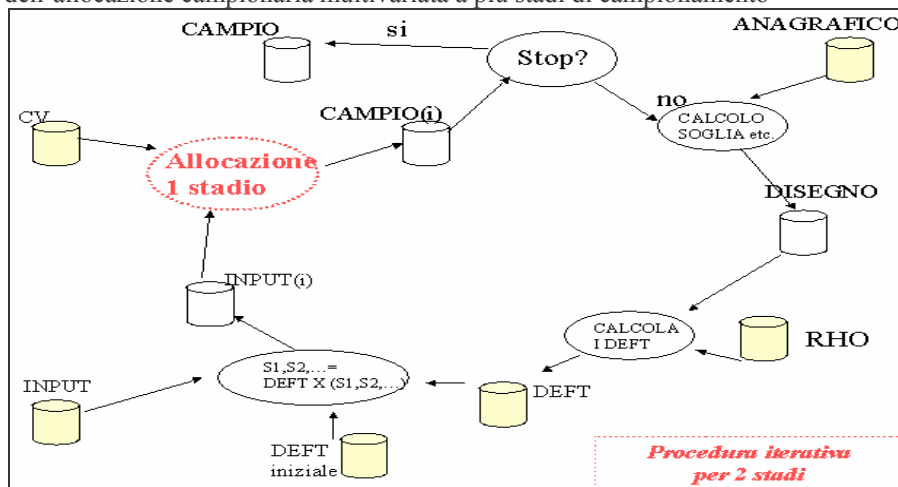
Figura 11: la procedura iterativa per adattare la procedura di calcolo dell'allocazione campionaria multivariata a più stadi di campionamento
