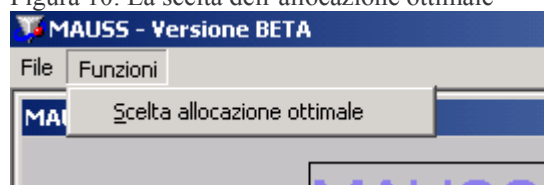
Figura 10: La scelta dell'allocazione ottimale
