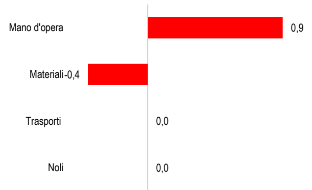
FIGURA 2. COSTO DI COSTRUZIONE DI UN FABBRICATO RESIDENZIALE. Contributi alla variazione tendenziale degli indici per gruppi di costo. Dicembre 2015, punti percentuali.
