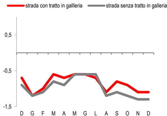
FIGURA 3. COSTO DI COSTRUZIONE DI TRONCHI STRADALI. Variazioni percentuali sullo stesso mese dell'anno precedente
