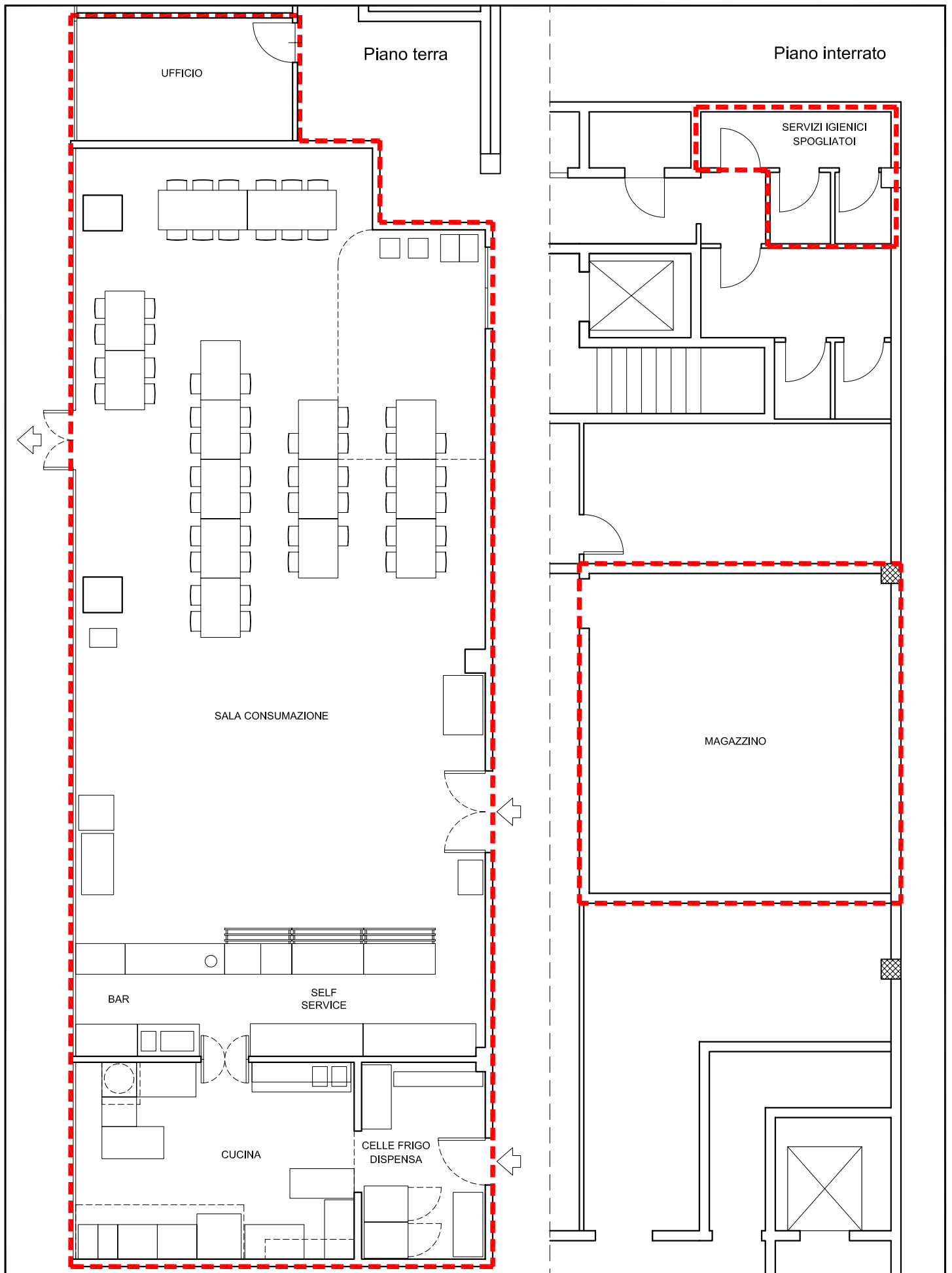
Planimetria piano terra e interrato: locali bar-mensa (scala 1:100)
